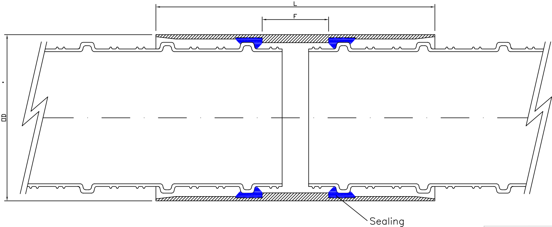
IP 4 PFS Coupler Dimensions
